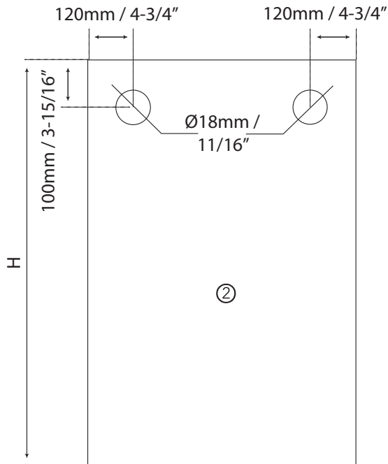
Corte del fijo del cristal
